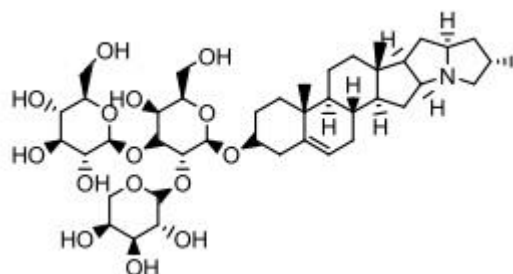
Gambar 4. Struktur saponin
