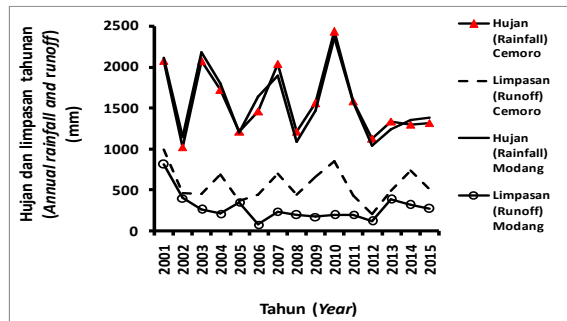
Gambar (Figure) 3. Hujan dan limpasan tahunan Sub DAS Cemoro dan Modang dari 2001 hingga 2015 (Annual rainfall and runoff Cemoro and Modang catchments from 2001 to 2015)
